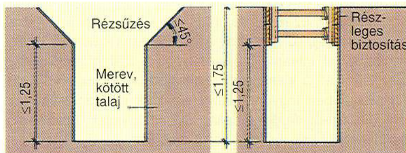
Falbiztosítás 1,25 m és 1,75 m közötti mélységű ároknál
