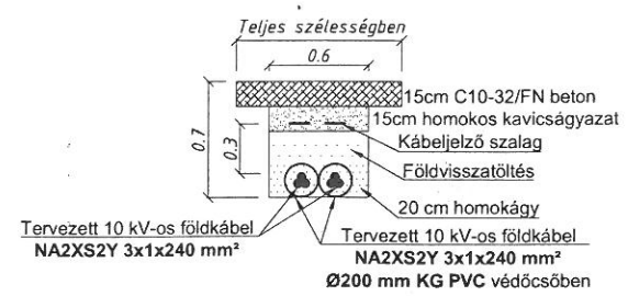
Kábelárok jellemző metszetrajza beton gépkocsibehajtóban M1:50
