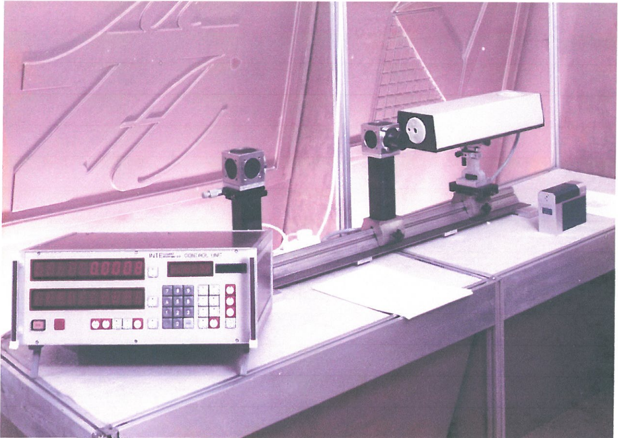
Lézer-interferométer mérőrendszer
